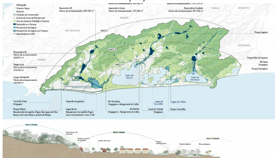
Figura 5 – Mapa geral de intervenções em Maricá e esquema de interpretação funcional espacial, de montante para jusante da bacia
