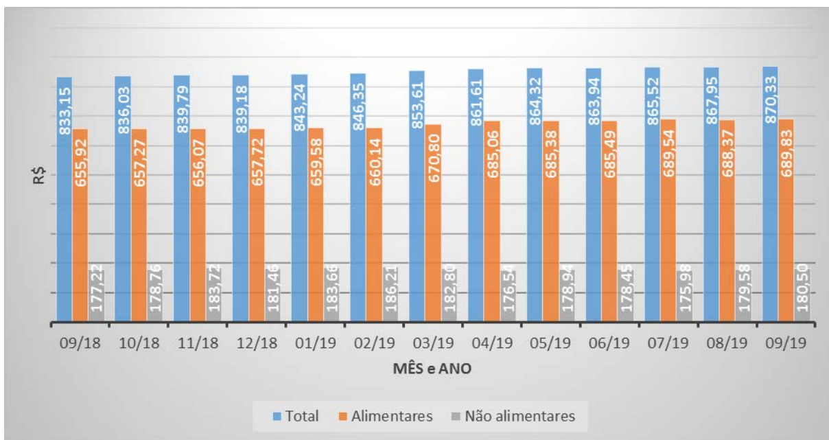
Figura 2: Evolução do custo com produtos alimentares e não alimentares da Cesta básica de Caxias do Sul de Setembro de 2018 a Setembro de 2019 (em R$)
