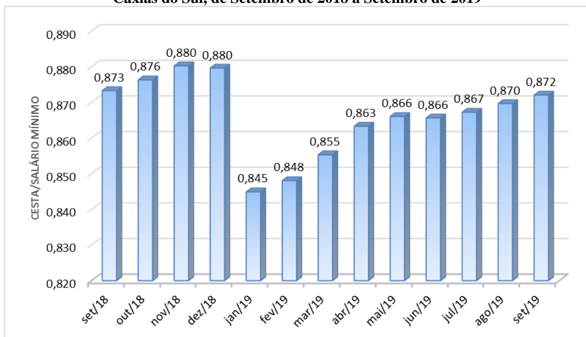
Figura 1: Quantidade de salários mínimos necessários para aquisição da Cesta básica de Caxias do Sul, de Setembro de 2018 a Setembro de 2019
