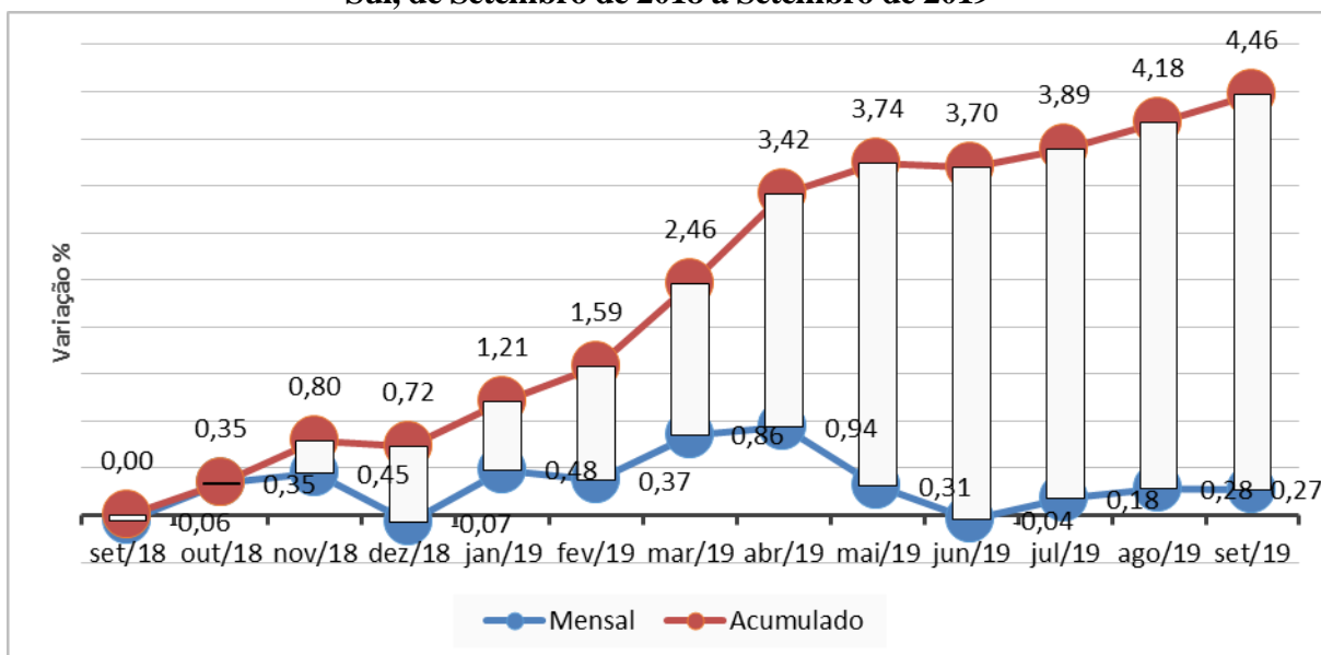
Figura 3: Variação percentual mensal e acumulada do custo da Cesta básica em Caxias do Sul, de Setembro de 2018 a Setembro de 2019
