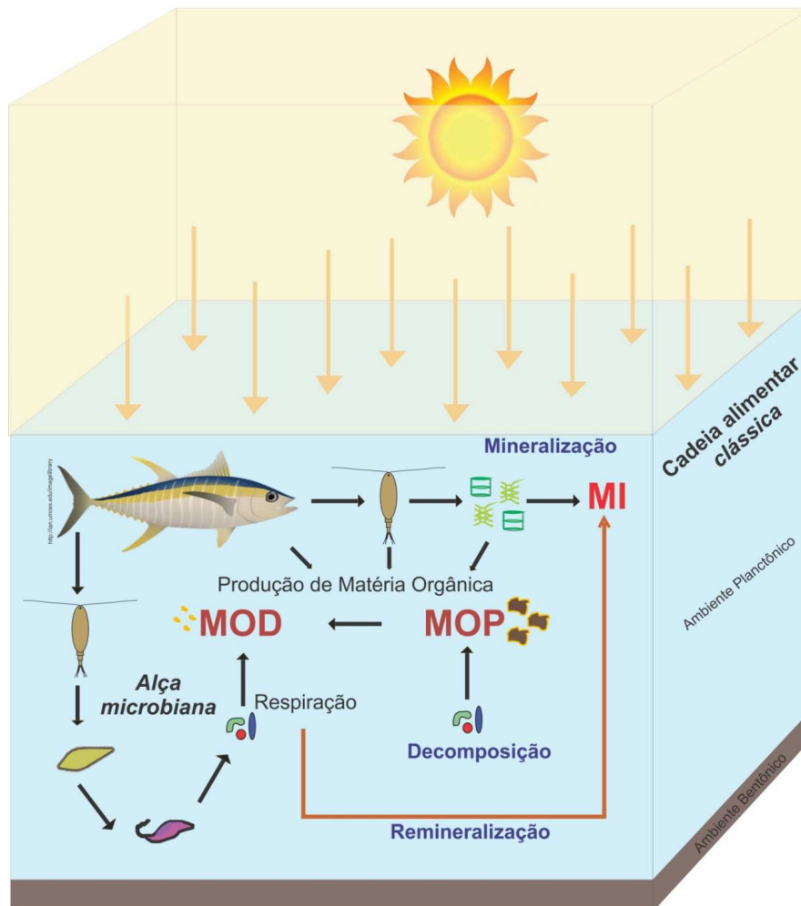
Figura 7 – Esquema representando a cadeia trófica marinha clássica e a alça microbiana, com ênfase nos processos de mineralização, remineralização e decomposição
