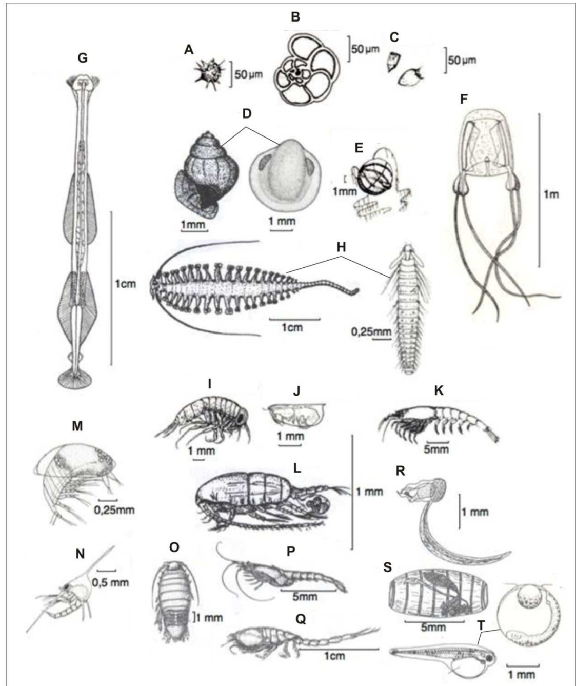
Figura 5 – Organismos zooplancônicos: A: Radiolaria; B: Foraminifera; C: Ciliata; D: Mollusca; E: Ctenophora; F: Cnidaria; G: Chaetognath; H: Polychaeta, I: Amphipoda; J: Ostracoda; K: Euphausiacea; L: Copepoda; M: Cirripedia; N: Decapoda; O: Isopoda; P: Misida; Q: Cumacea; R: Appendicularia (Larvacea); S: Doliolida; T: Chordata
