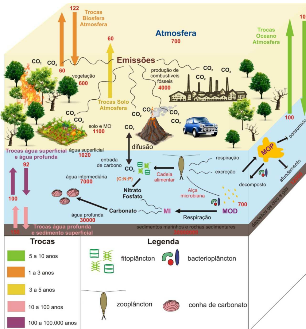
Figura 8 – O ciclo do Carbono, com reservas e trocas entre reservatórios. Valores em bilhões de toneladas (Gt) de Carbono
